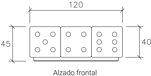
Alzado frontal
