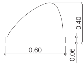
Alzado lateral
