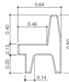
Alzado lateral
