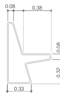
Alzado lateral
