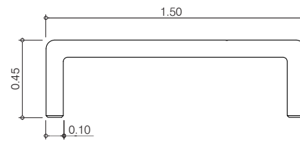
Alzado frontal
