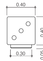
Alzado lateral
