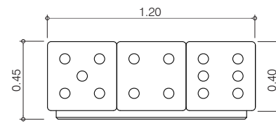
Alzado frontal
