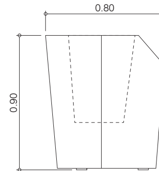
ALZADO
