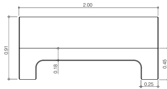
Alzado frontal
