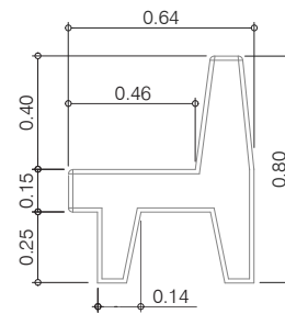
Alzado lateral
