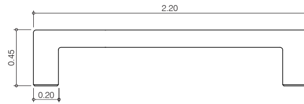
Alzado frontal
