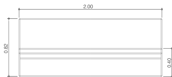
Alzado frontal
