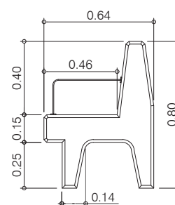
Alzado lateral
